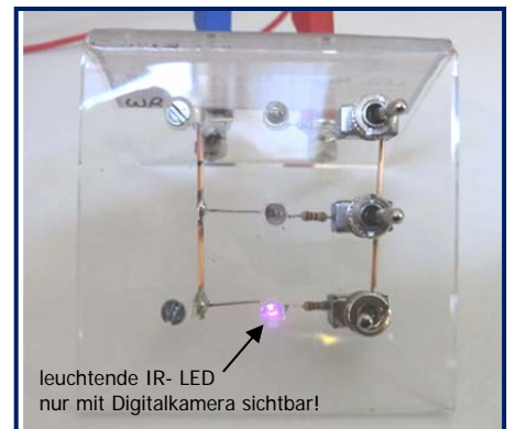
Nur die IR- LED ist angeschaltet, die Digitalkamera/ Smartphone- Kamera zeigt das IR- Licht violett an, mit dem Auge ist das Leuchten nicht sichtbar.
