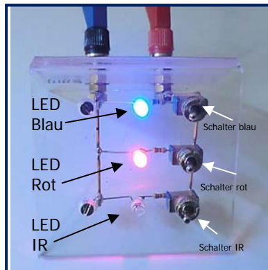
Die eingeschalteten 3 LED's, oben blau, in der Mitte rot, unten das IR- Licht, für das menschliche Auge unsichtbar, sichtbar mit einer Digitalkamera
