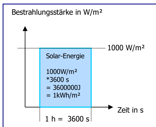
Abb.4: Eingestrahlt Solar-Energie bei einer Bestrahlungsstärke von 1000\text{ W/m}^2 und einer Zeitdauer von 1\text{ h} = 3600\text{ s}
