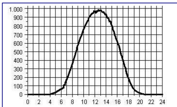
Abb.5: Tagesverlauf einer Bestrahlungsstärke in \text{W/m}^2 (y- Achse) von 0 – 24 Uhr (x- Achse) an einem wolkenlosen Sommertag (Quelle: NILS-ISFH). Das Messmodul SUSE 5.23/5.23A ist auf einem Süddach mit 35^\circ Dachneigung montiert.
